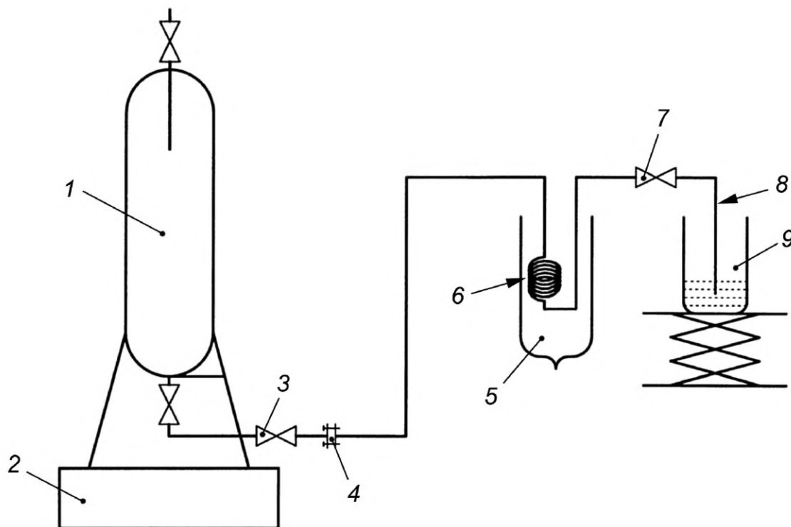
1 — баллон с образцом по 6.1; 2 — весы с точностью измерения до 1 г (6.14.1); 3 — V-образный игольчатый клапан, пропускающий сжиженный углеводородный газ в линию (6.8.2); 4 — опора проходного фильтра (6.2 и 6.3); 5 — сосуд Дьюара, заполненный по 6.5; 6 — охлаждающий змеевик из нержавеющей стали (6.4); 7 — игольчатый клапан (6.8.1); 8 — трубка из ПТФЭ длиной 20 см; 9 — лабораторный неглубокий стакан (6.9) вместимостью 5 дм 3 , содержащий 50 см 3 дихлорметана (5.4)
