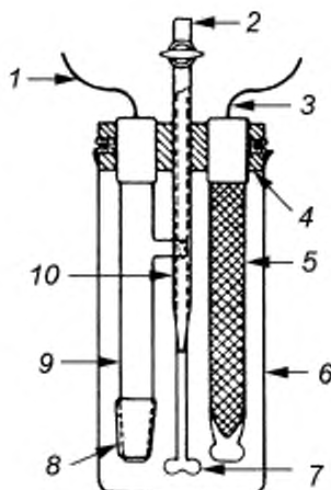
1 — провод к халомельному стеклянному электроду; 2 — бюретка E; 3 — экранированный провод к стеклянному электроду; 4 — бакелитовая опора; 5 — стеклянный индикаторный экран; 6 — стакан A; 7 — пролеллерная мешалка (за кончиком бюретки) D; 8 — муфта (пришлифованное соединение); 9 — халомельный электрод сравнения B; 10 — удлиненный кончик бюретки (перед мешалкой)
