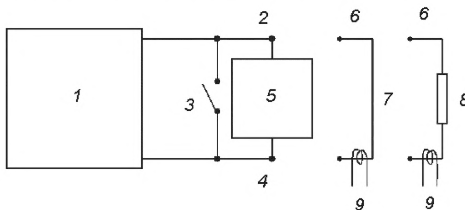
1 — генератор ЭСР импульсов по МЧТ (номинально 200 пФ/1,5кОм); 2 — вывод А; 3 — переключатель; 4 — вывод Б; 5 — образец; 6 — оценочная нагрузка; 7 — закорачивающий провод; 8 — сопротивление 500 Ом; 9 — преобразователь тока
