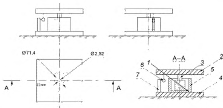
1 — образец; 2, 4 — нижняя и верхняя плиты пресса; 3 — круглый штамп; 5 — емкость для испытания; 6 — индикатор, 7 — стойка
