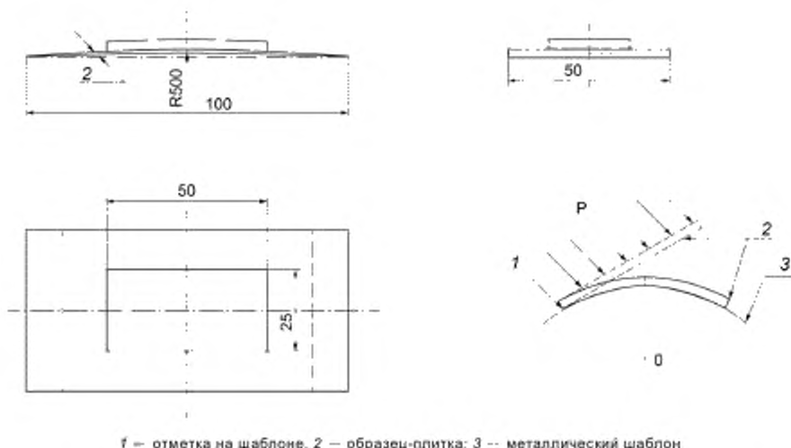
1 — отметка на шаблоне, 2 — образец-плитка; 3 — металлический шаблон
