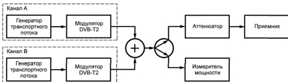
Рисунок 3 — Схема проверки 3
