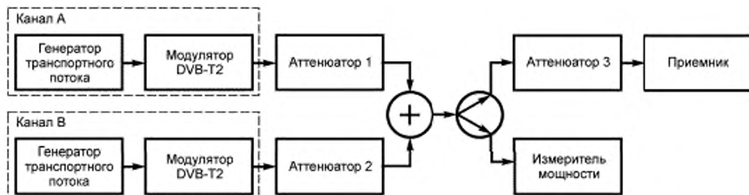
Рисунок 4 — Схема проверки 4
