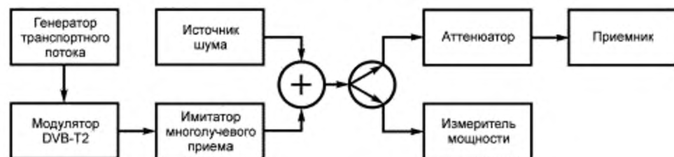
Рисунок 2 — Схема проверки 2
