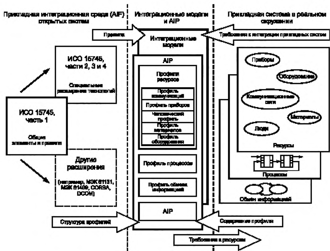
Рисунок 1 — Область применения комплекса стандартов ИСО 15745
