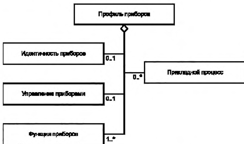
Рисунок 12 — Диаграмма класса общего профиля приборов
