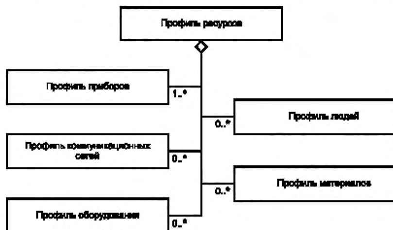
Рисунок 10 — Диаграмма общего класса профиля ресурсов
