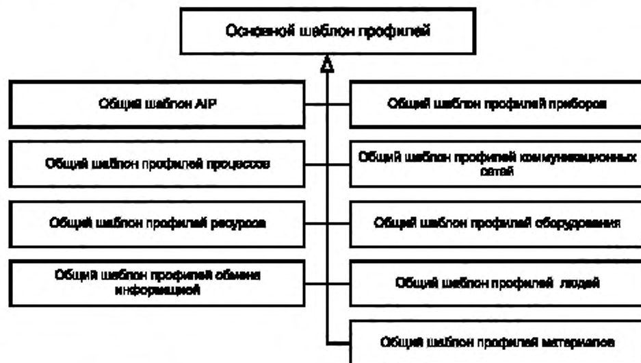
Рисунок 3 — Диаграмма классов основного/общего шаблонов профилей
