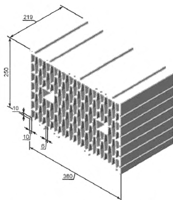
Рисунок А.1.21 — Камень крупноформатный 10,7 НФ
