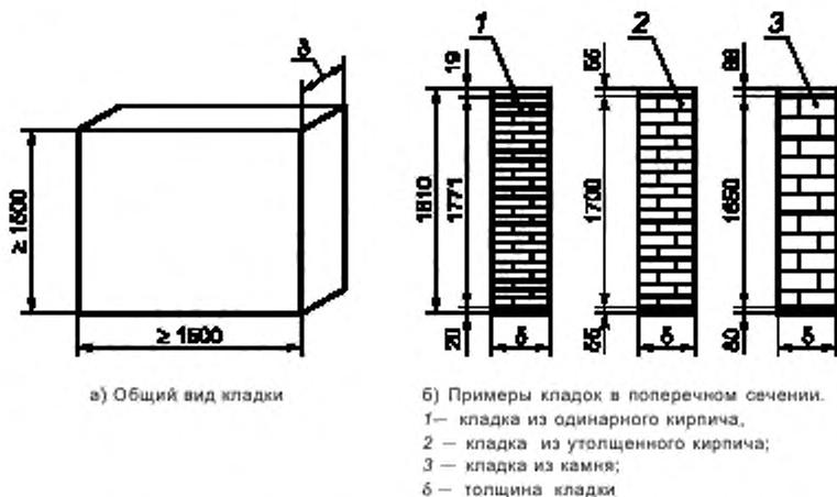
Рисунок 2 — Фрагмент кладки для определения теплопроводности
