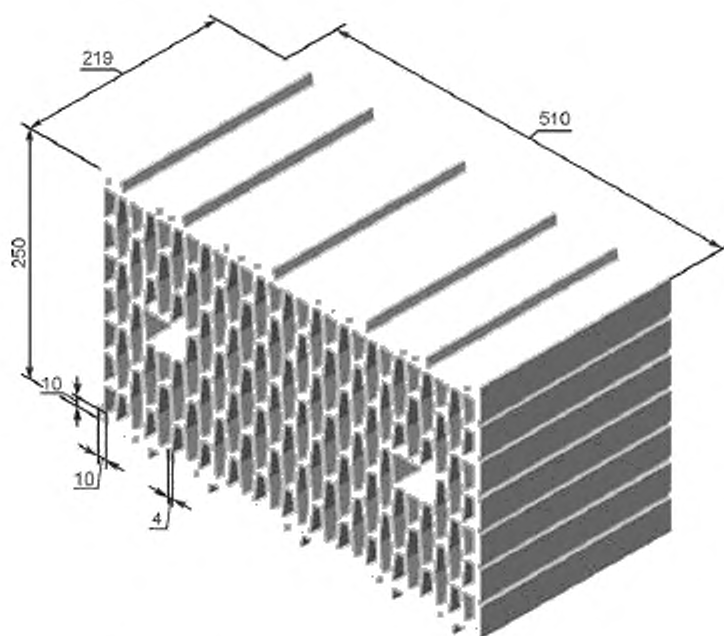
Рисунок А.1.23 — Камень крупноформатный 14,3 НФ
