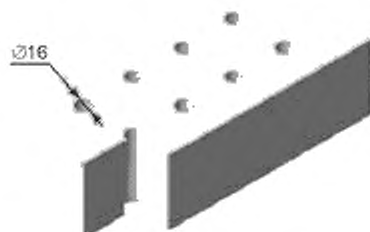
Рисунок А.2.3 — Кирпич формата 1 НФ с восемью цилиндрическими отверстиями
