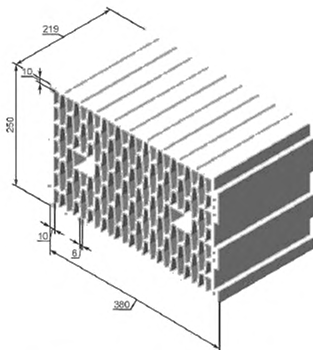
Рисунок А.1.22 — Камень крупноформатный 10,7 НФ
