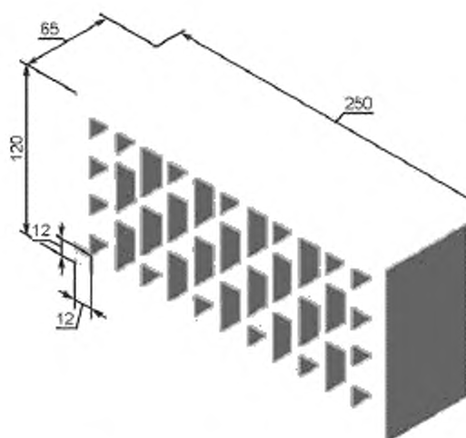
Рисунок А.1.9 — Кирпич формата 1 НФ с 35 пустотами
