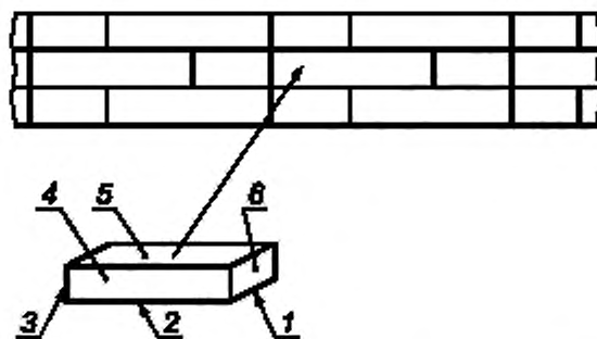
1 — ширина; 2 — длина; 3 — толщина; 4 — ложок; 5 — постель; 6 — тычок
