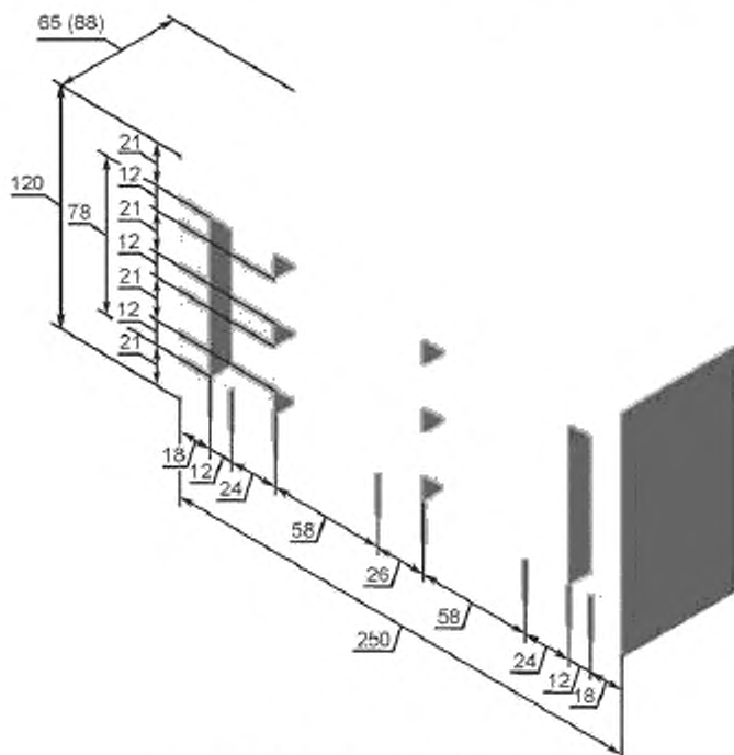
Рисунок А.1.3 — Кирпич формата 1(1,4) НФ с восемь щелевидными пустотами
