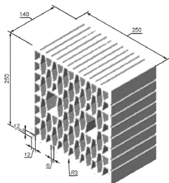
Рисунок А.1.20 — Камень крупноформатный 4,5 НФ
