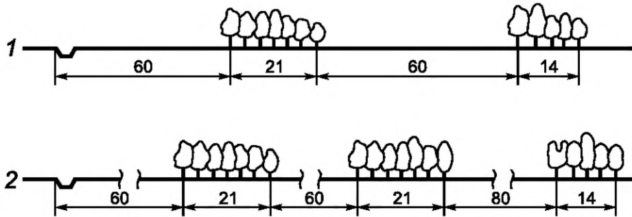
Рисунок 2 — Схемы снегозащитных насаждений для объемов снегоприноса более 300 м 3 /м
