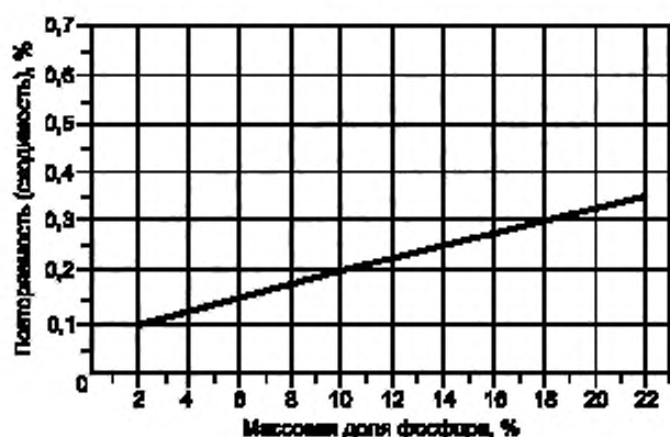
Рисунок 2 — Повторяемость (сходимость) гравиметрического метода
