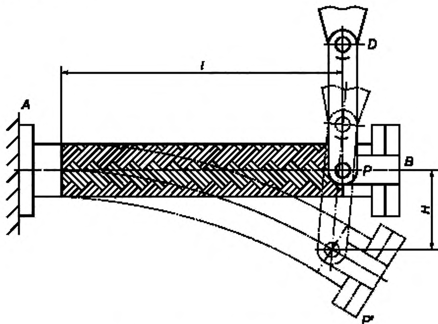
Рисунок 2 — Монтаж гибкого шланга в приспособление
