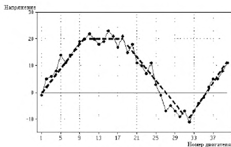
в) Cusum-карта
