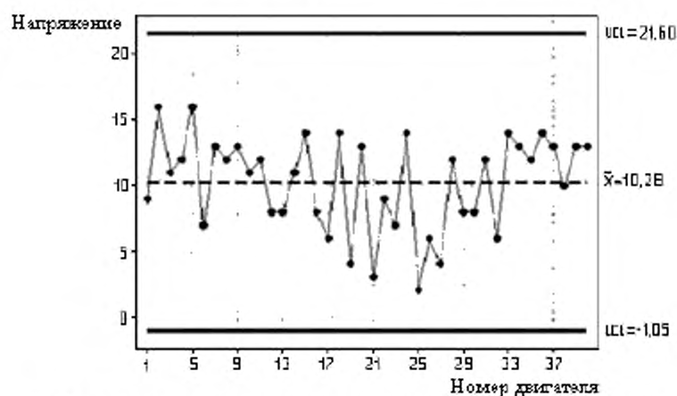
б) Стандартная контрольная карта индивидуальных значений
