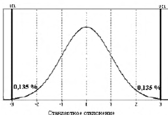
Рисунок 4 – График плотности нормированного нормального распределения
