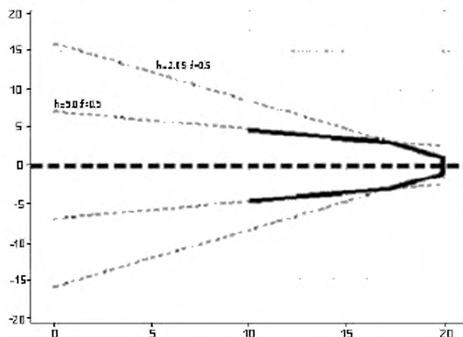
Рисунок 10 – Усеченная V-маска
