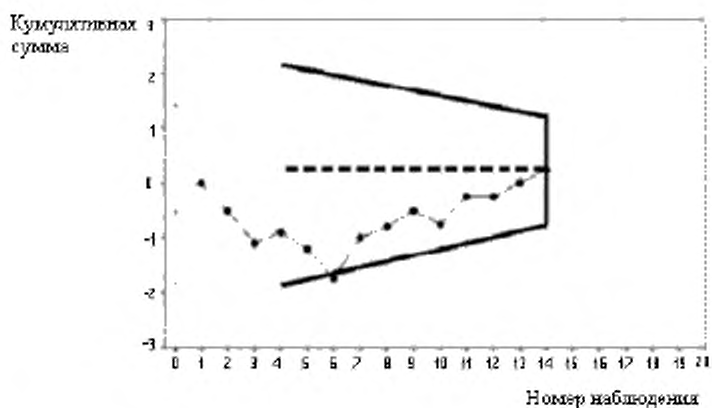
Рисунок 7 – Примеры использования усеченной V-маски для обнаружения существенного изменения среднего процесса
