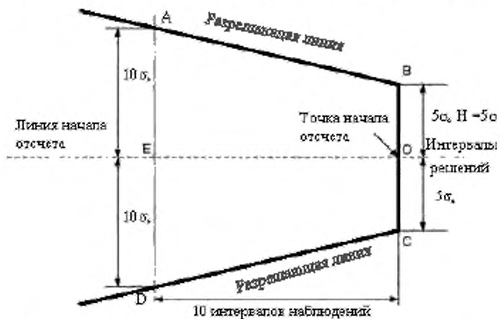
Рисунок 5 – Форма и размеры усеченной V-маски общего назначения
