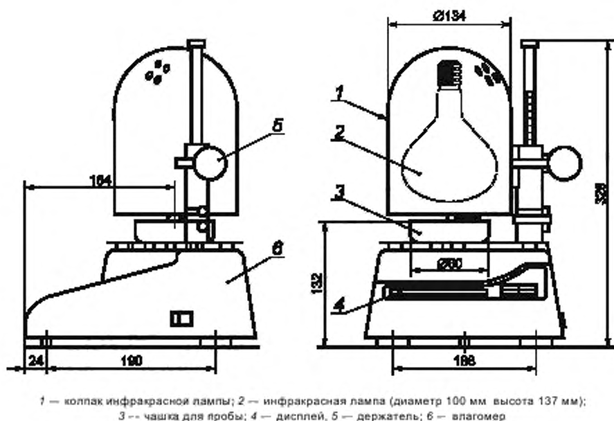
Рисунок 1 — Пример инфракрасного влагомера
