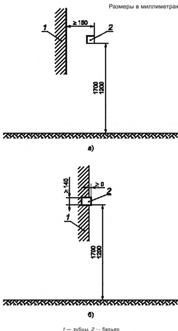
Рисунок 4 — Расположение барьера при хранении машины
