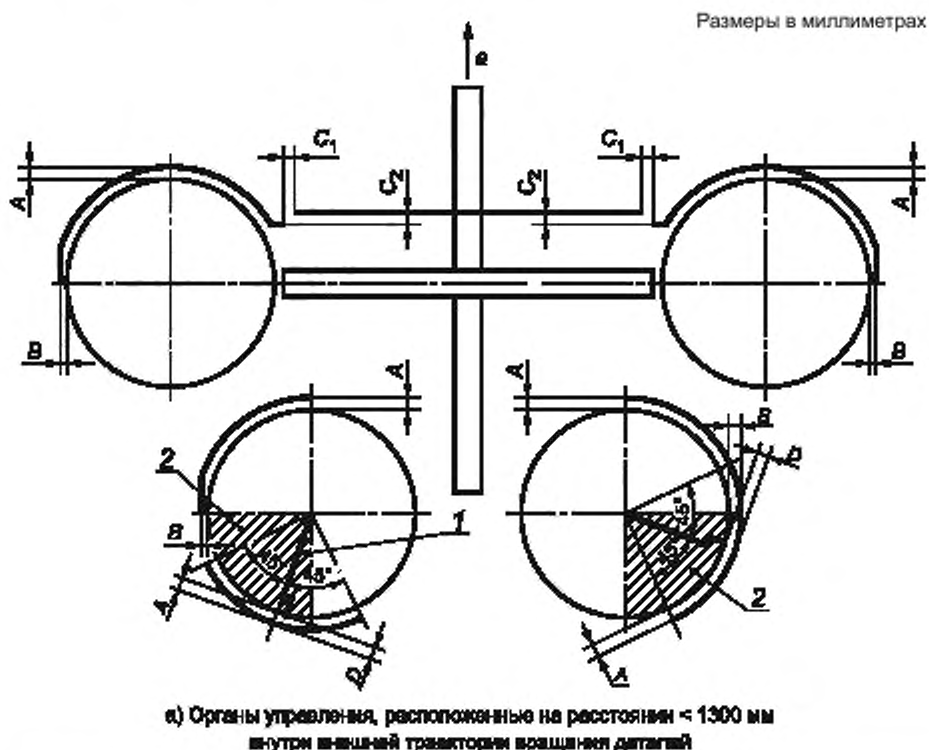
Рисунок 3, лист 1 — Защитные приспособления на роторах при расположении органов управления позади задних роторов
