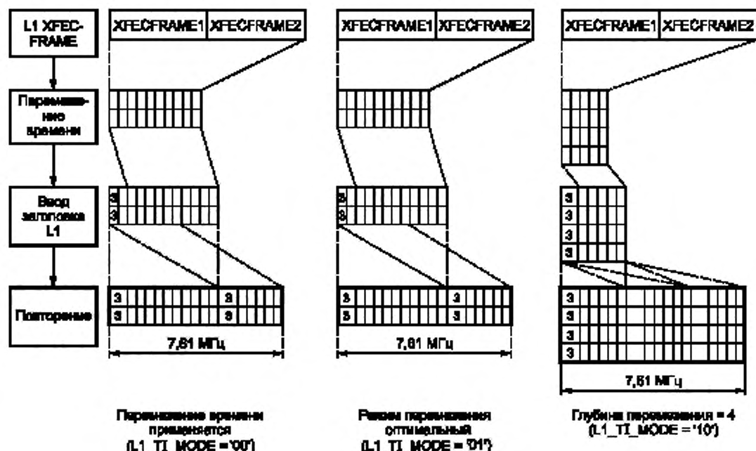
Рисунок 31 — Перемеживание времени данных сигнализации L1-part2
