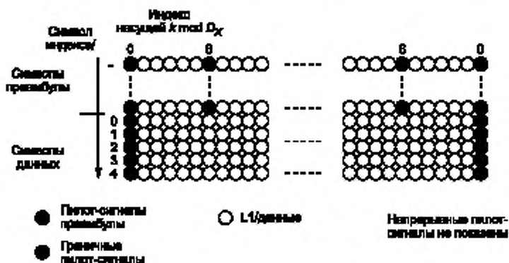
Рисунок 41 — Расположение граничных пилот-сигналов в спектре OFDM сигнала
