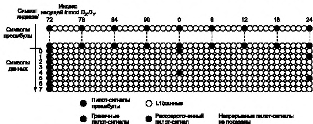
Рисунок Е.8 — Рассредоточенный пилот-сигнал для GI 1/128 с низкочастотной границей k \bmod D_x D_y = 72
