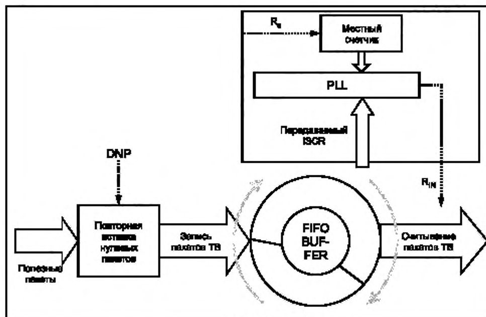
Рисунок Д.1 — Пример блок-схемы приемника повторной вставки пакетов и синхронизации восстановленной тактовой частоты R_{TS}
