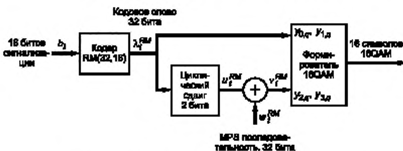
Рисунок 21 — Заголовок FECFrame высокой производительности
