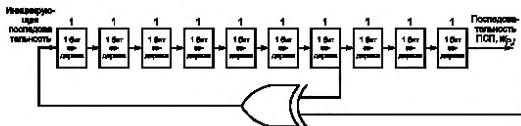
Рисунок 35 — Схема генератора ПСП для модуляции пилот-сигналов
