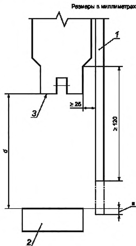
1 — защитное приспособление; 2 — неподвижная часть пресс-подборщика; 3 — крайнее нижнее положение кривошипа; a \geq 0 если d < 300
