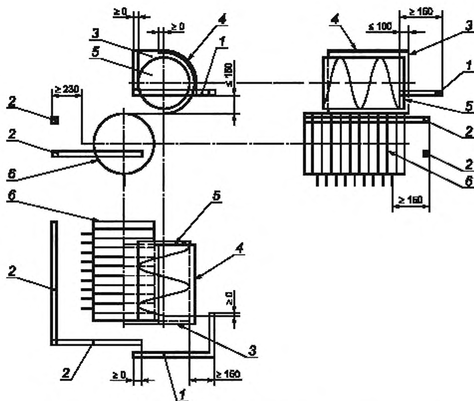
1 — ограждение; 2 — ограждение, согласно 5.2.2.1; 3 — боковое неподвижное защитное приспособление; 4 — задняя крышка над шнеком; 5 — загрузочный шнек; 6 — подборщик
