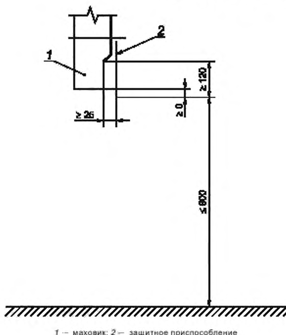
Рисунок 4 — Защита маховика
