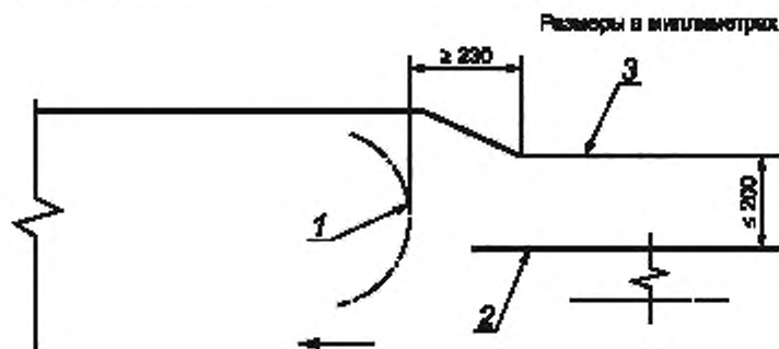
1 — задний внешний контур обвязывающего механизма; 2 — верх прессовальной камеры; 3 — защитное приспособление
