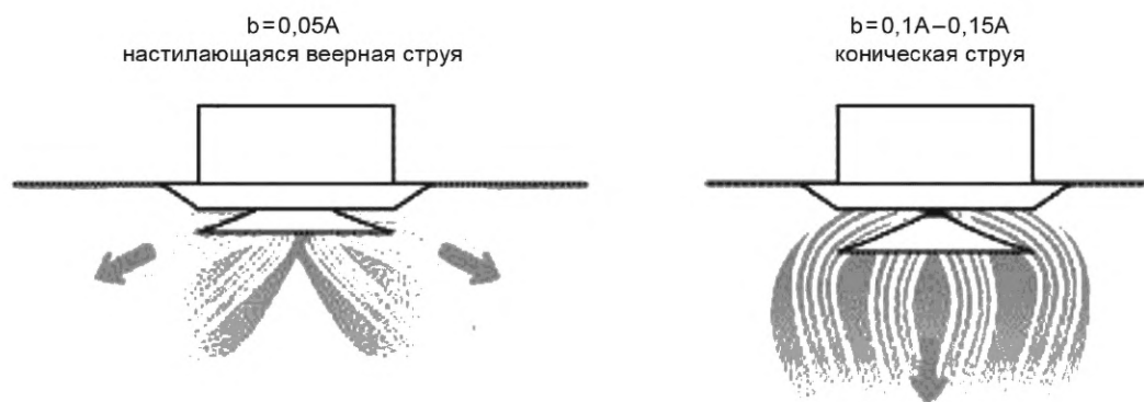
Рисунок 2 — Схемы струй, формируемых диффузором
