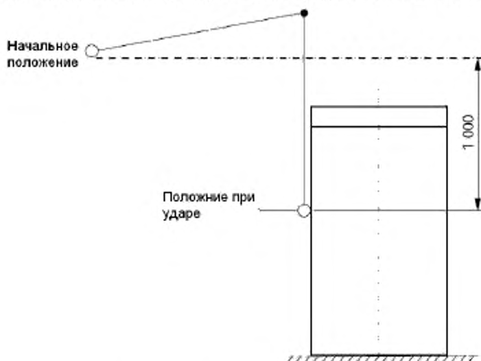
Рисунок 103а — Схема проведения испытания для подтверждения стойкости к удару при монтаже НКУ-ОП-Д на земле зафиксированным в предназначенном основании
