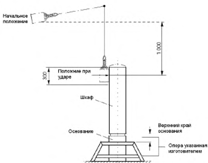
Рисунок 102a — Схема проведения испытания для подтверждения стойкости к ударной нагрузке при монтаже НКУ-ОП-Д на земле зафиксированным в предназначенном основании
