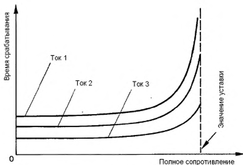
Рисунок 5 — Время срабатывания в нормальных условиях
