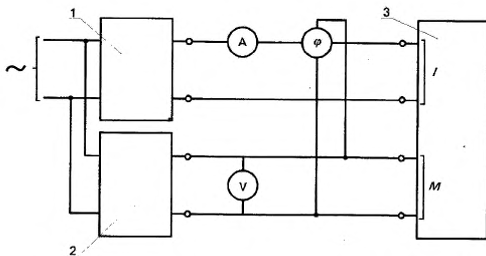
1 — регулируемый источник тока; 2 — регулируемый источник напряжения со сдвигом фаз от 0 до 360^\circ ; 3 — испытуемое реле
