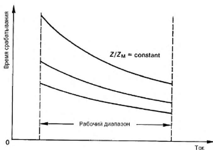
Рисунок 5 — Время срабатывания в нормальных условиях
