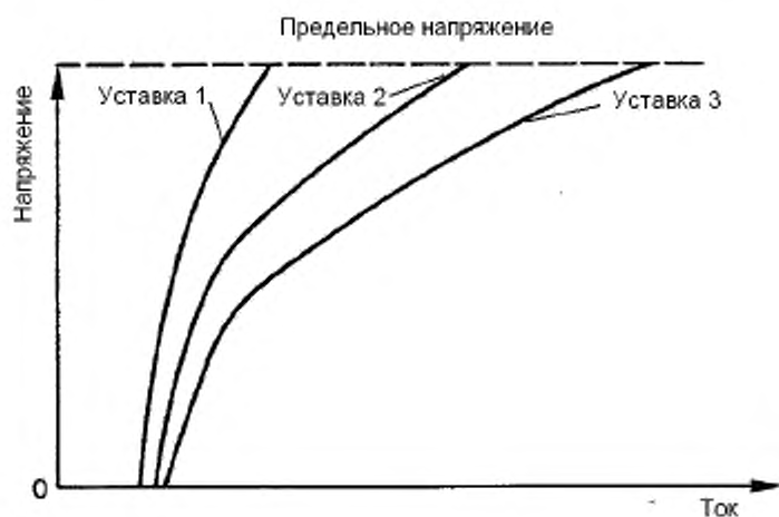
Рисунок 3 — Характеристика срабатывания U = f(I)
