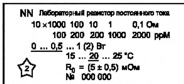
Рисунок 3 — Пример маркировки пятидекадного резистора
