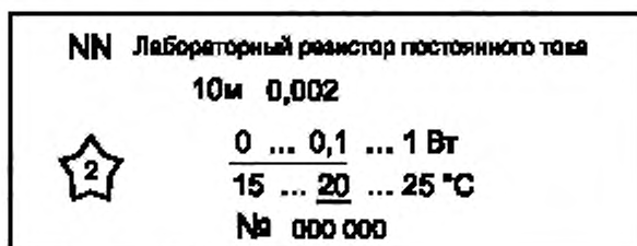
Рисунок 2 — Пример маркировки единичного резистора
