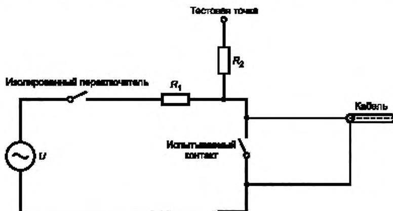
Рисунок D.1 — Схема для кабельной нагрузки
