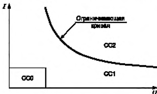
Рисунок С.3 — Категории контактных нагрузок
