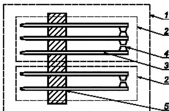
Рисунок А.2 — Пример объяснения терминов по контактам
