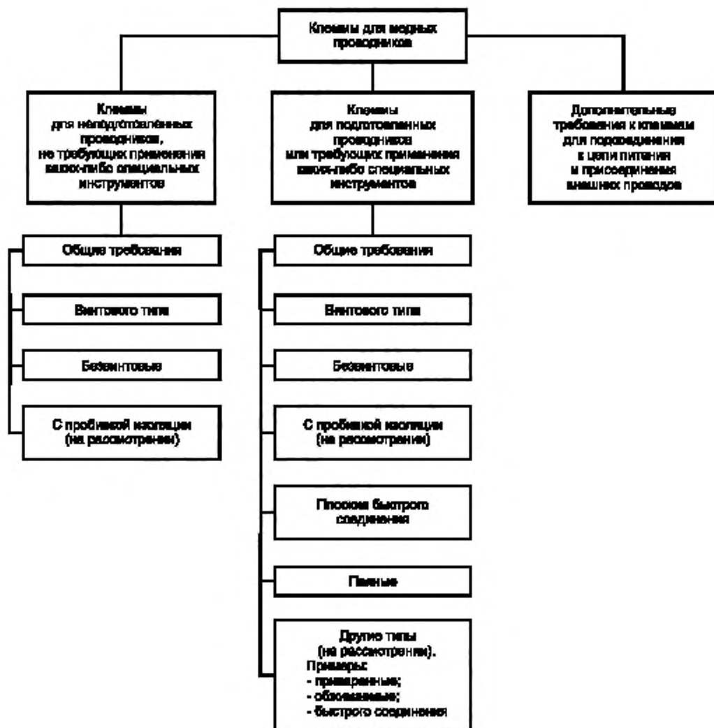
Рисунок J.1 — Схема семейств клемм
