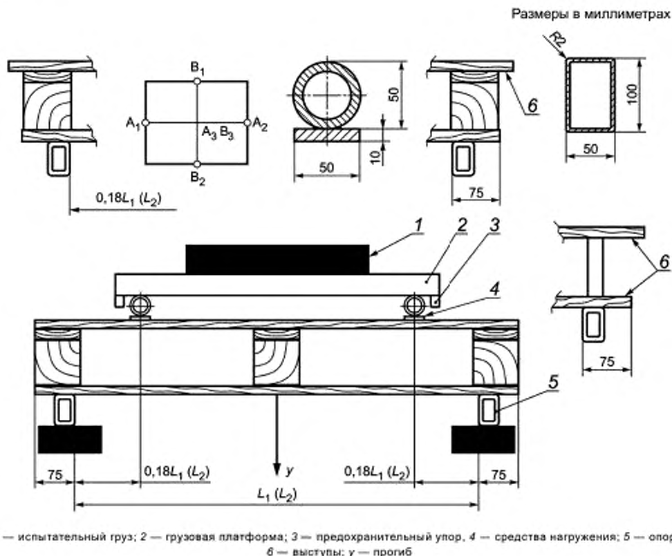
Рисунок 1 — Испытание на изгиб
