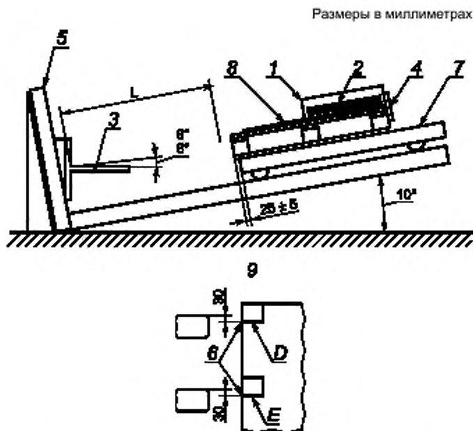
1 — коробка с грузом; 2 — испытательный груз; 3 — ударный упор, 4 — съемный упор для коробки с грузом; 5 — задний упор; 6 — точки соударения; 7 — тележка; 8 — лист распределения нагрузки; 9 — вид сверху; L — расстояние между точкой соударения и положением, в котором тележку отпускают
