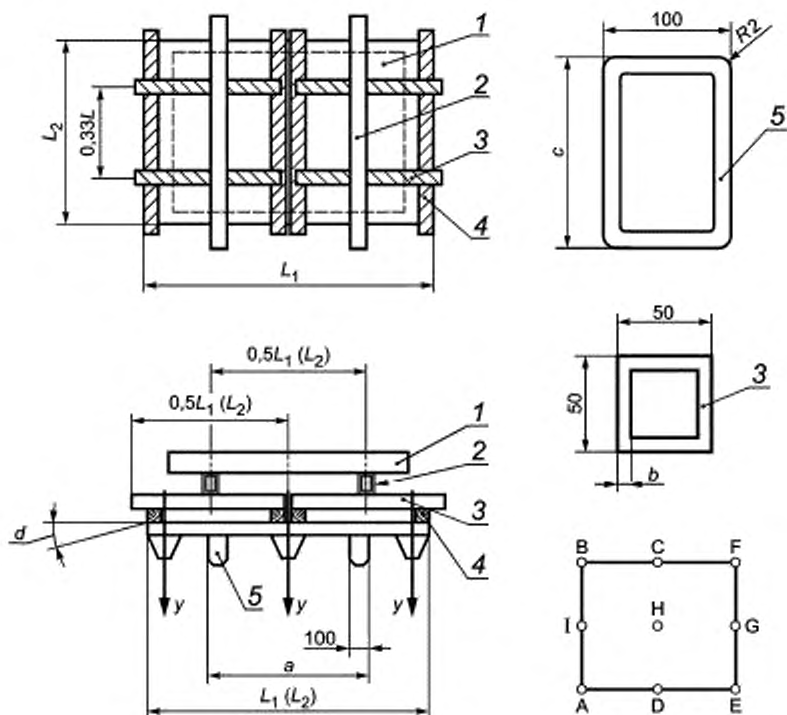
1 — испытательная нагрузка, 2 — средства нагружения; 3 — стальной брусок — груз 50 \times 50 \text{ мм} \times L (> \frac{1}{2} L_1) ; 4 — стальной брусок — груз 50 \times 50 \text{ мм} \times (> L) ; 5 — опора; A и I — точки измерения прогиба; y — прогиб; a — расстояние между опорами 570 мм или 690 мм; b — толщина стального бруска — груза > 3 \text{ мм} ; c — длина опоры до 200 мм; d — угол прогиба настила поддона при испытании
