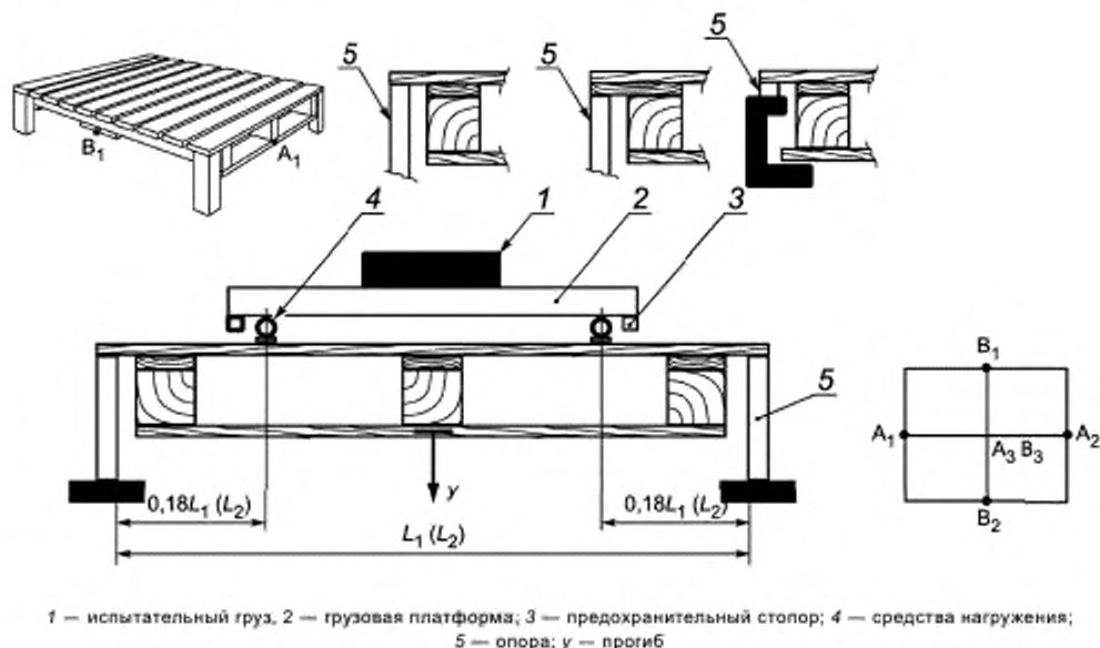
Рисунок 6 — Испытание на изгиб поддона с выступами
