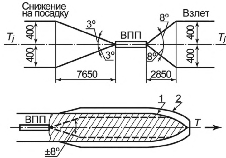
T — регламентируемый интервал времени (см. приложение А); T_j — регламентируемый интервал времени для j -го типа ВС; 1 — контур шума, построенный для взлета самолета по идеальной прямой; 2 — то же с учетом отклонения от идеального маршрута полета
