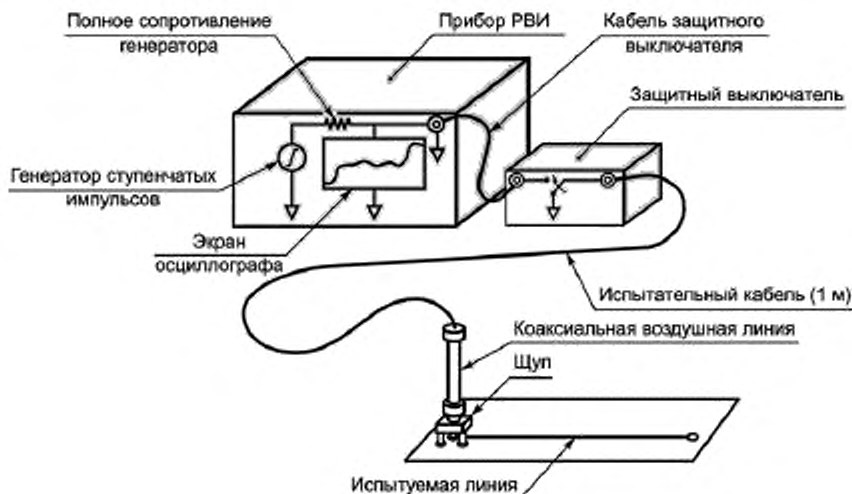
Рисунок 18 — Вариант схемы испытания
