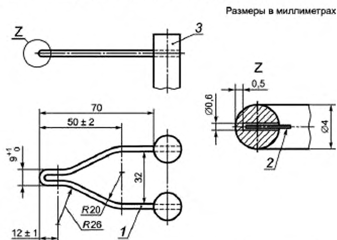
Рисунок 1 — Раскаленная проволока
