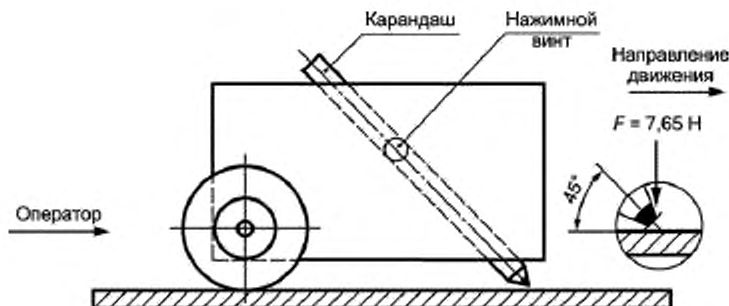
Рисунок 14 — Держатель карандашей
