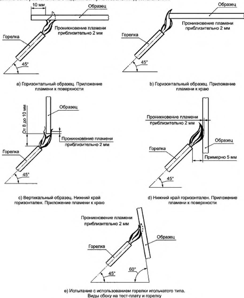
Рисунок 3 — Испытание с использованием горелки игольчатого типа
