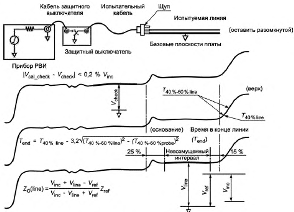
Рисунок 19 — Неискаженный интервал
