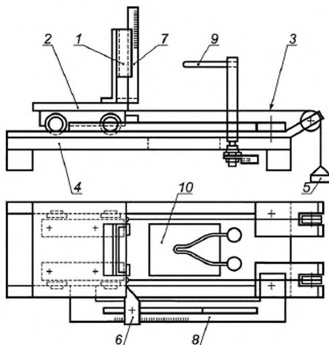
Ключ: 1 — установочный зажим; 2 — каретка; 3 — натяжной шнур; 4 — плита основания; 5 — груз; 6 — упор; 7 — шкала для измерения пламени; 8 — шкала проникновения; 9 — раскаленная проволока (см. рисунок 1); 10 — сквозное отверстие в плите основания для частиц, падающих с образца.
