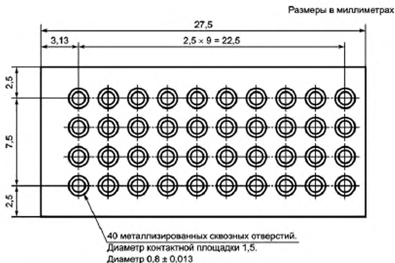
Рисунок 30 – Рекомендуемый образец для испытания металлизированных сквозных отверстий
