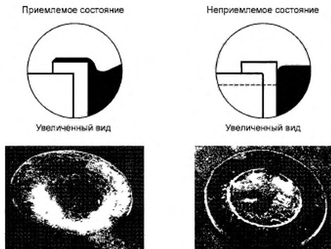
Рисунок 32 — Качество смачивания металлизированных сквозных отверстий припоем
