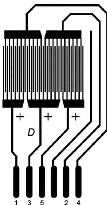
Рисунок 28 — Типовой рисунок «Гребенка»
