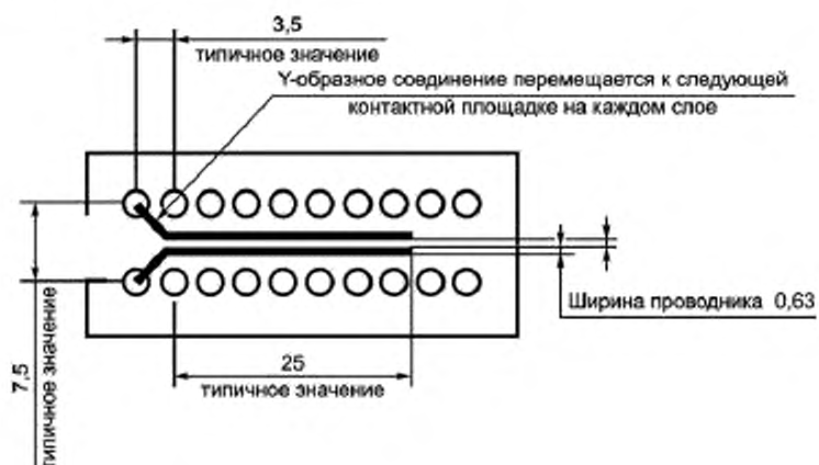
Рисунок 27 — Купон для испытания на сопротивление изоляции, мкм
