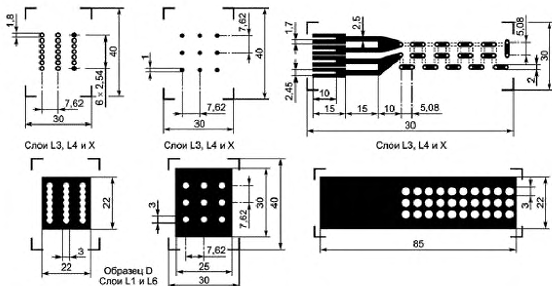
b) Расположение образцов для испытания
