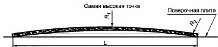
Рисунок 8 — Схема проведения измерения изгиба
