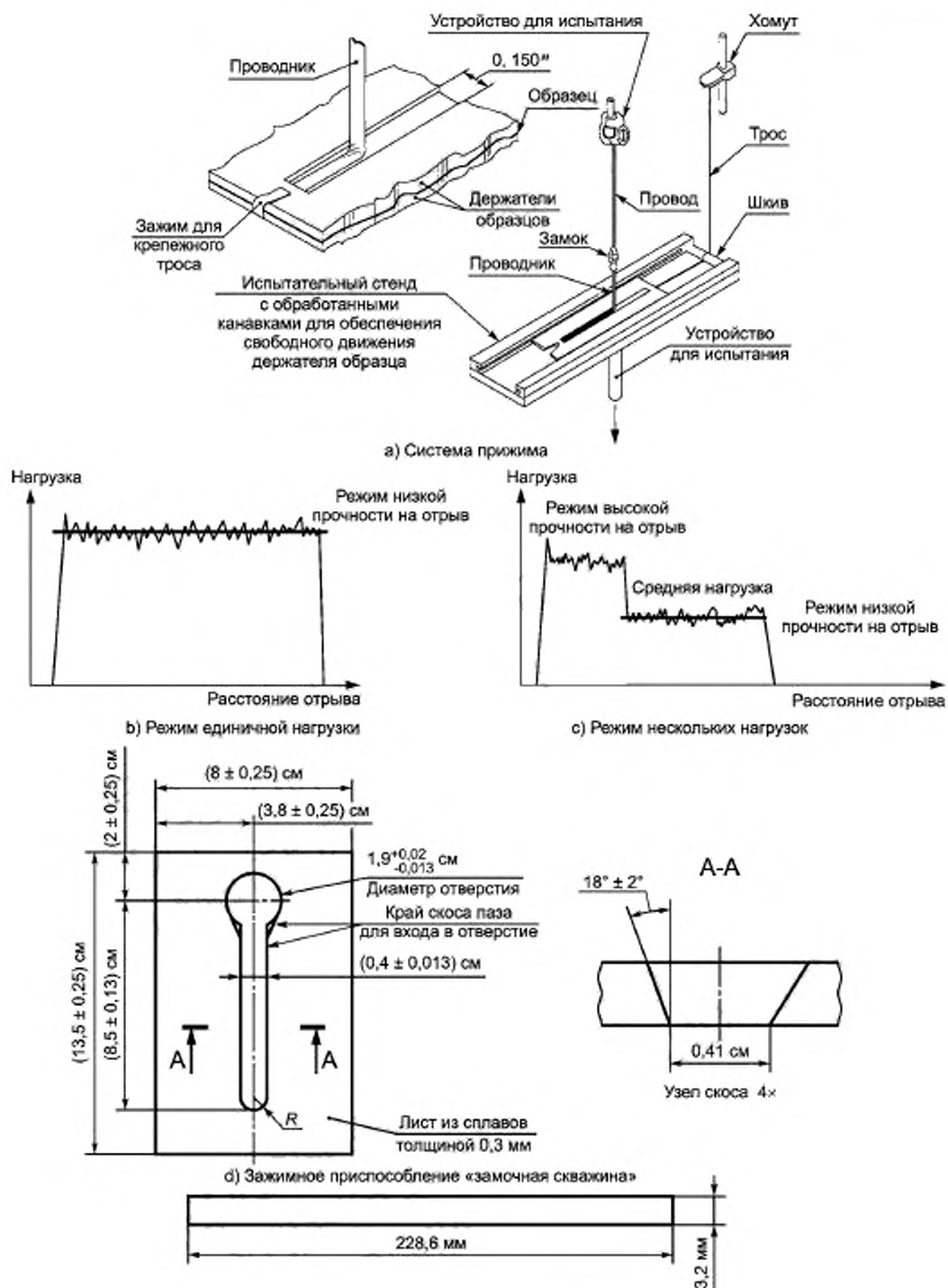
Рисунок 5 — Медная фольга для испытания на отрыв
