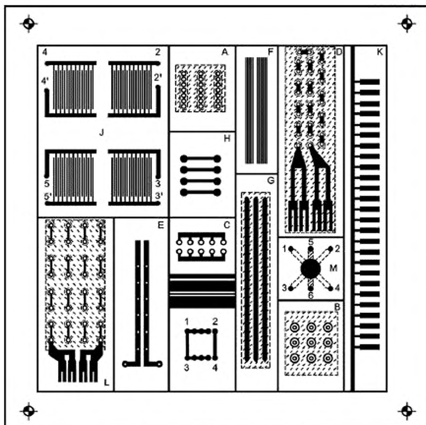
а) Расположение образцов для испытания
