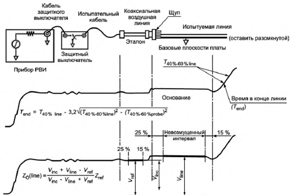
Рисунок 20 — Пример формы испытательного сигнала
