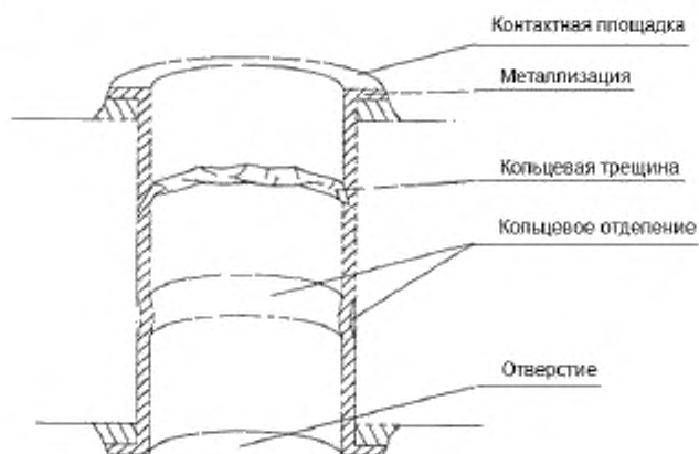
Рисунок 2 – Кольцевые дефекты
