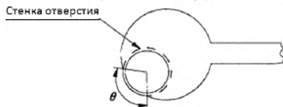
Рисунок 5 – Минимальная ширина W_2 кольца внутренней контактной площадки
