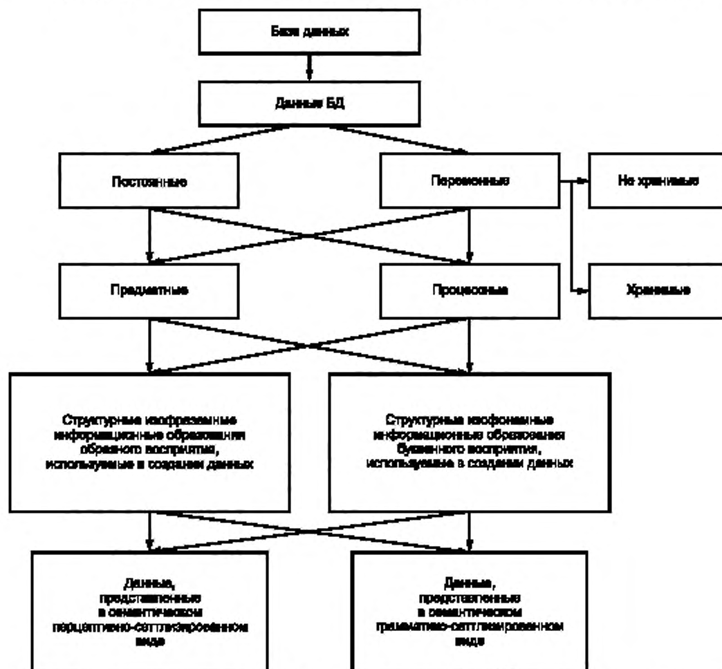
Рисунок Б.1 — Схема структуры данных в БД, разрабатываемой с применением ноон-технологии (вариант)
