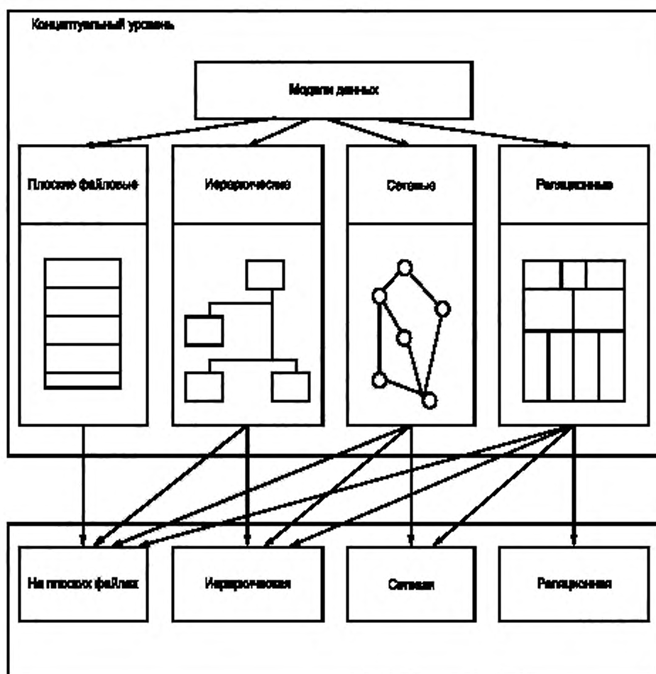
Рисунок В.1 — Схема отображения моделей данных основными типами СУБД
