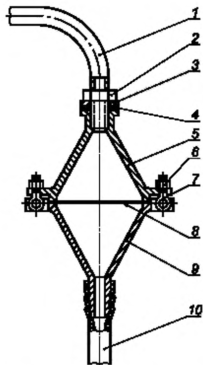
1 — трубка соединительная; 2, 6 — лайка; 3 — шайба, 4 — прокладка; 5, 9 — крышка; 7 — пикт. 8 — фильтр, 10 — трубка резиновая
