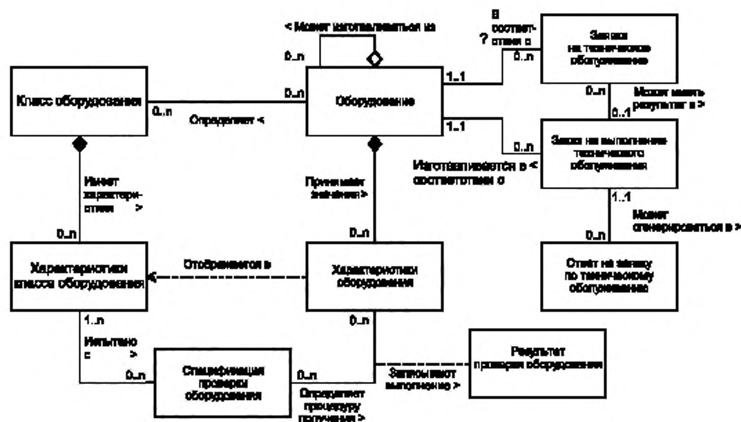
Рисунок 3 — Модель оборудования
