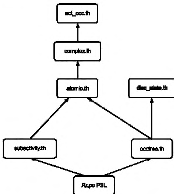
Рисунок 1 — Зависимости между наборами аксиом внешнего ядра PSL
