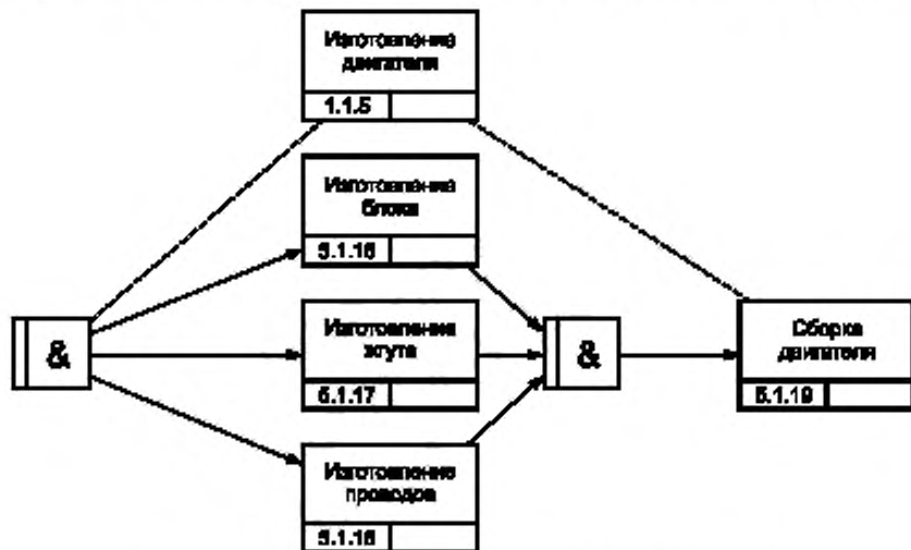
Рисунок С.2 — Процесс изготовления двигателя 350-Engine
