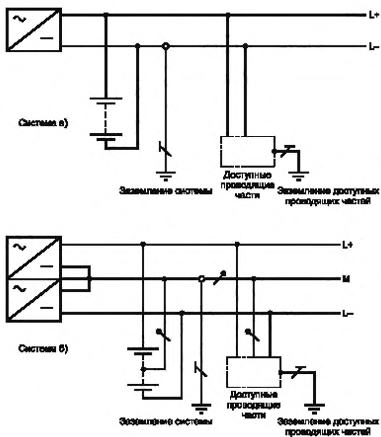
Рисунок Б.8 — ТТ система постоянного тока
