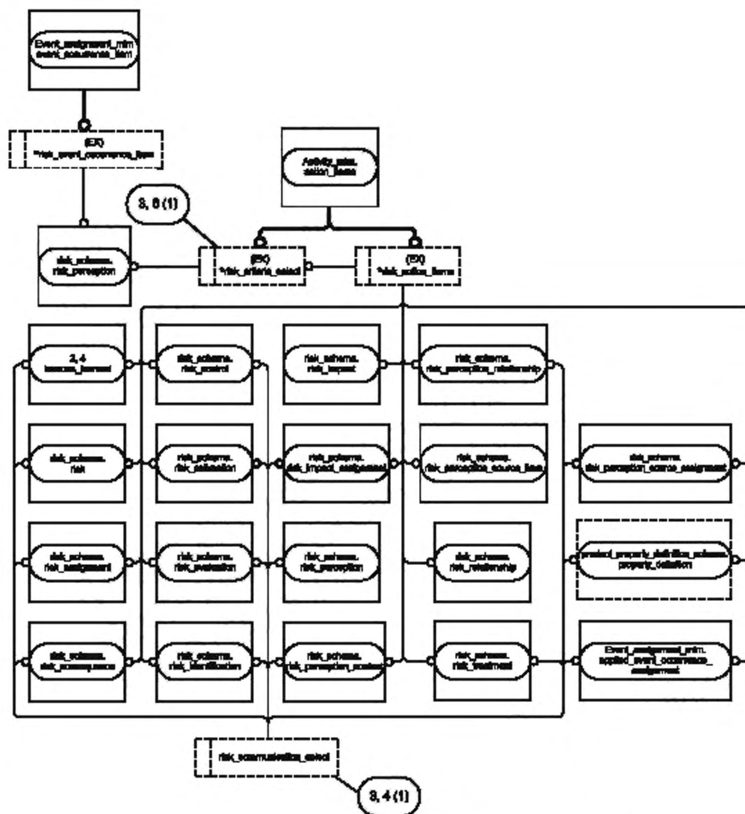
Рисунок D.4 — Представление ИММ на уровне объектов в формате EXPRESS-G (диаграмма 3 из 3)
