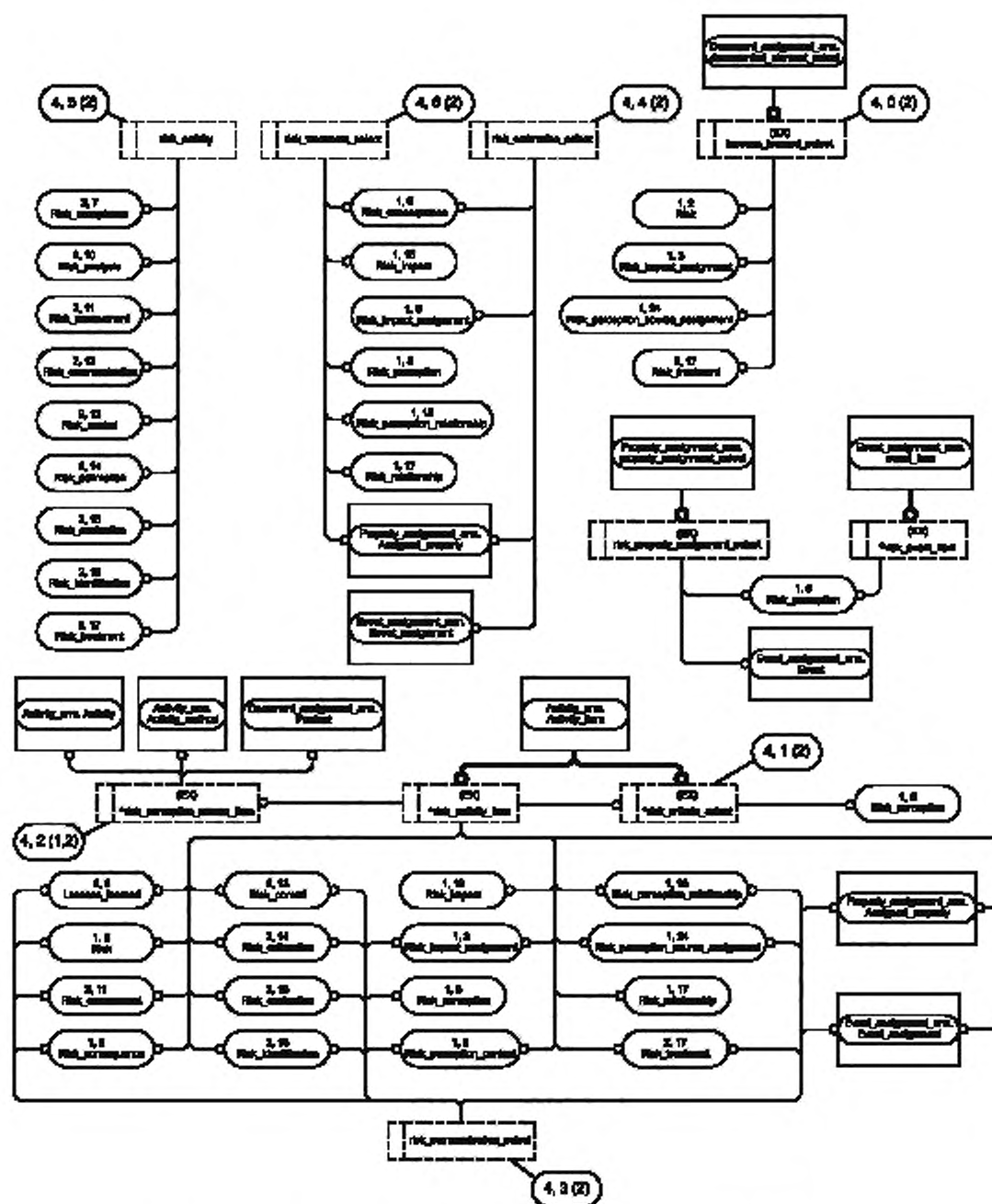
Рисунок С.5 — Представление ПЭМ на уровне объектов в формате EXPRESS-G (диаграмма 4 из 4)
