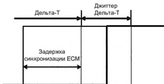
Рисунок 5 — Временная диаграмма джиттера Дельта-Т Figure 6:
