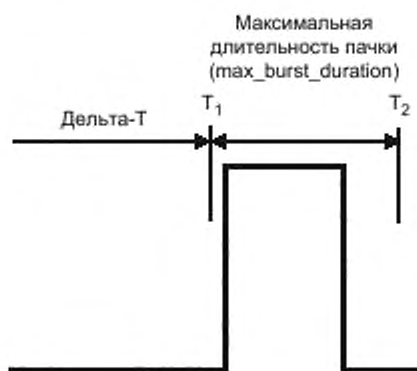
Рисунок 7 — Максимальная длительность пачки
