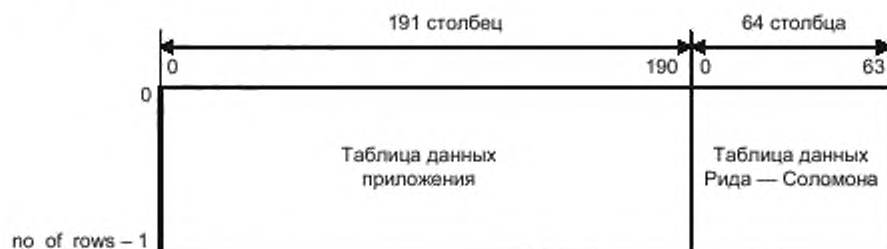
Рисунок 8 — Структура кадра MPE-FEC
