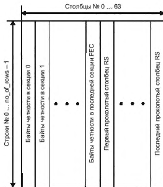
Рисунок 11 — Схема таблицы данных Рида — Соломона
