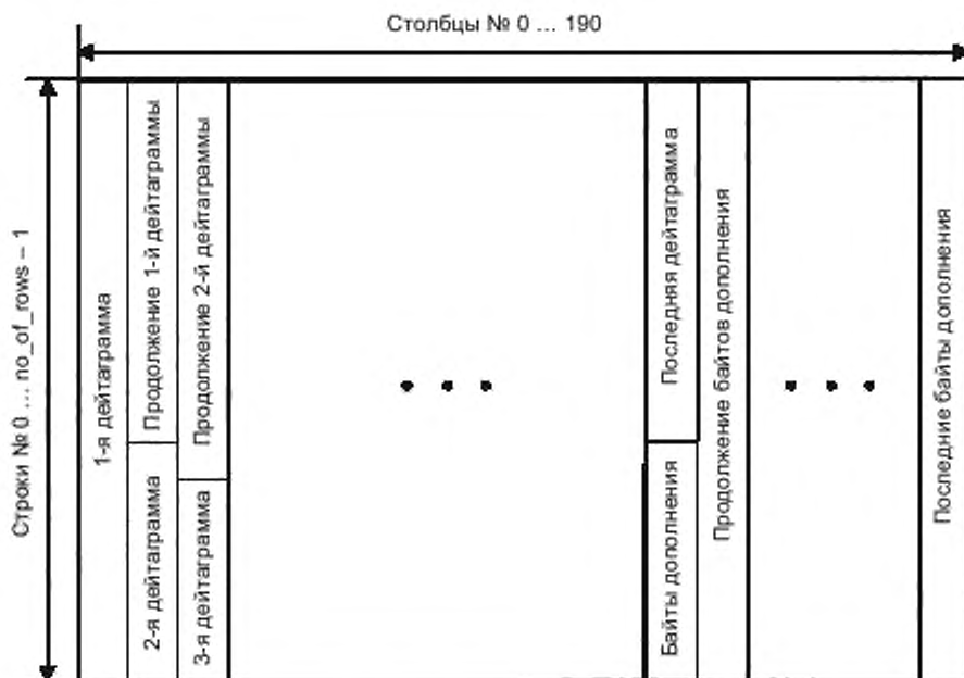
Рисунок 10 — Схема таблицы данных Приложения
