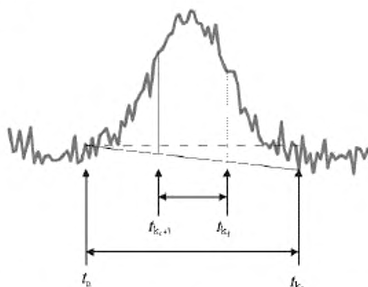
Рисунок 4 – Модели наложения выше горизонтальной линии (пунктирная линия) и наклонной линии (сплошная линия) между точками t_{k+1} и t_{k_2}
