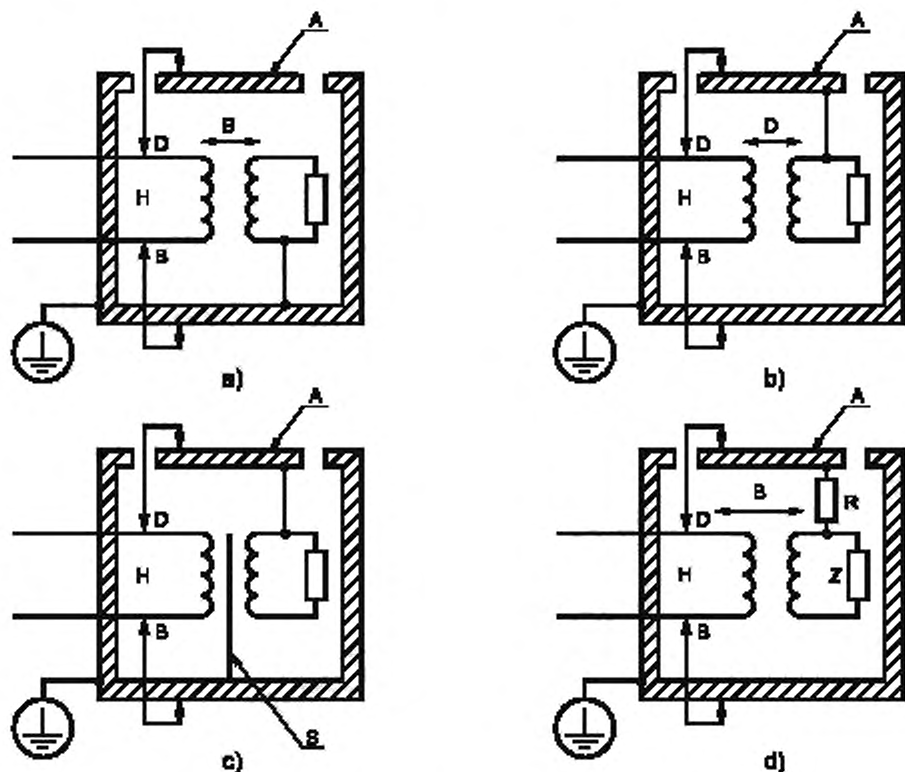
Рисунок D.1 а) — d) — Защита между опасными для жизни и доступными частями
