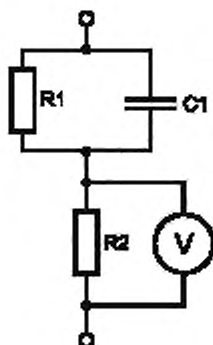
Рисунок А.4 — Схема измерения тока при влажном контакте
