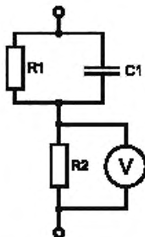
Рисунок А.3 — Схема измерения тока, вызывающего электрические ожоги
