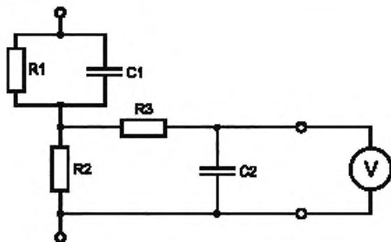
Рисунок А.1 — Схема измерения переменного тока при частоте до 1 МГц и постоянного тока
