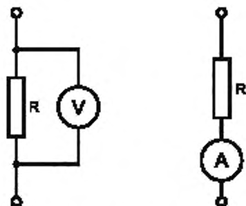
Рисунок А.2 — Схемы измерения переменного тока напряжением синусоидальной формы при частотах до 100 Гц и напряжения постоянного тока
