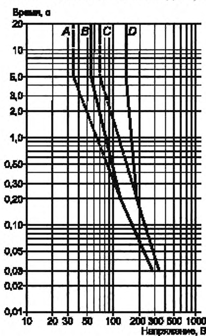
Рисунок 2 — Максимальная длительность кратковременных доступных напряжений при условии единичной неисправности (см. 6.3.2, перечисление а))
