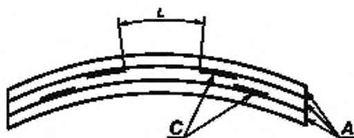
L — расстояние между соседними проводниками; A — слой тонкопленочного материала, например ленты полиэфирной пленки; C — проводники
