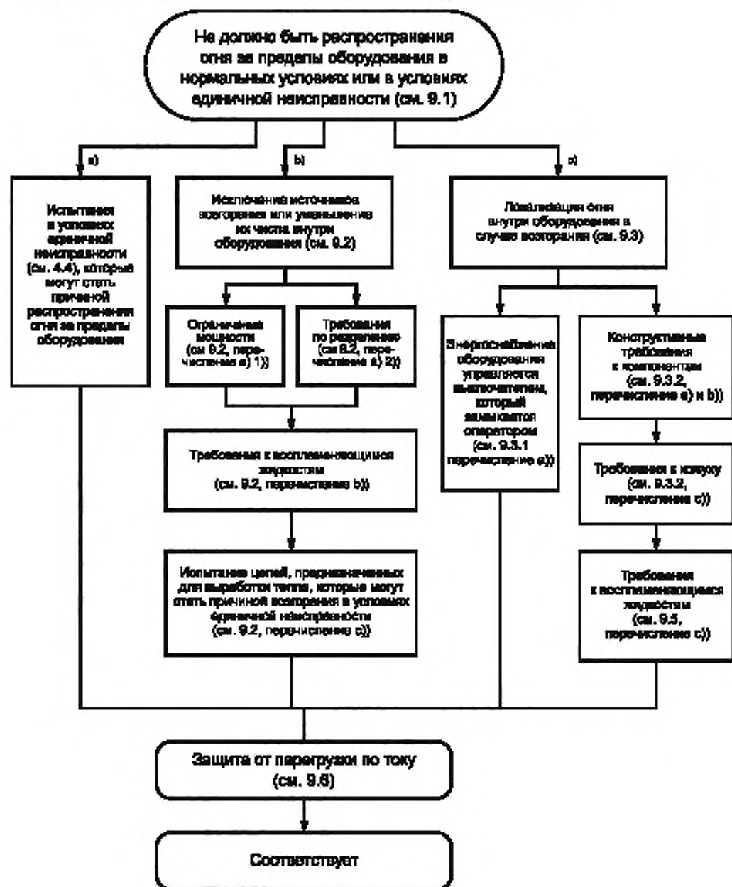
Рисунок 11 — Схема требований к защите от распространения огня
