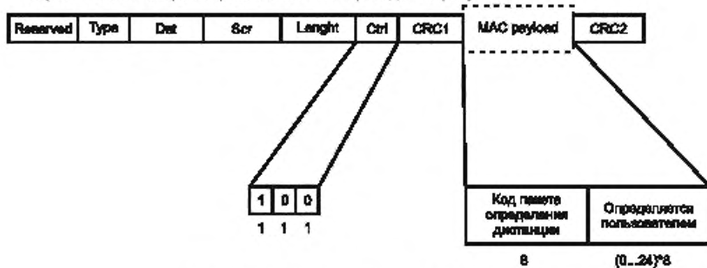
Рисунок 54 – Формат пакета измерения расстояния T4R1
