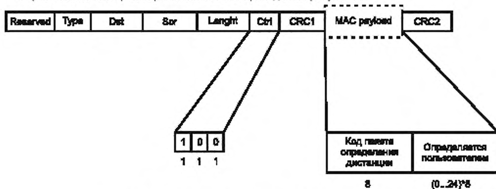
Рисунок 52 – Формат пакета измерения расстояния T3R1
