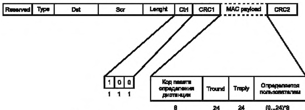
Рисунок 51 – Формат пакета измерения расстояния T2R3
