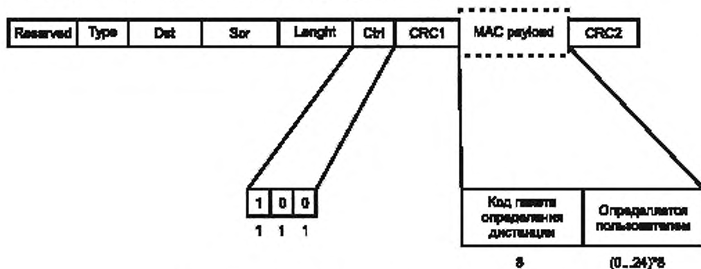
Рисунок 50 – Формат пакета измерения расстояния T2R2
