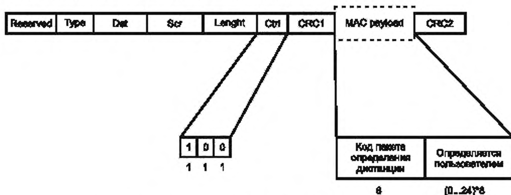
Рисунок 49 – Формат пакета измерения расстояния T2R1
