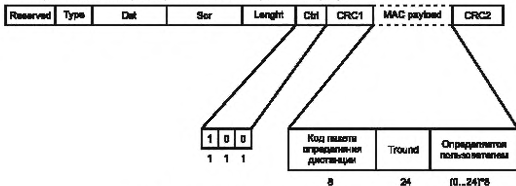
Рисунок 55 – Формат пакета измерения расстояния T4R2
