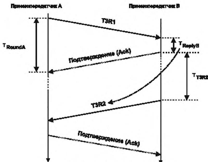
Рисунок 58 – Обмен пакетами измерения расстояния типа 3
