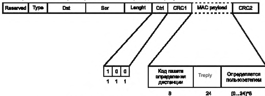
Рисунок 53 – Формат пакета измерения расстояния T3R2
