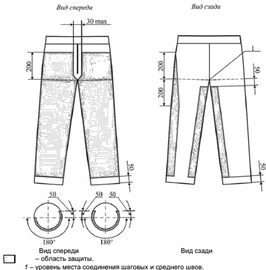
Рисунок 2 – Конструкция В
