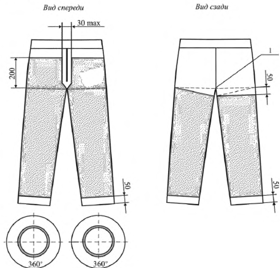
Рисунок 3 – Конструкция С
