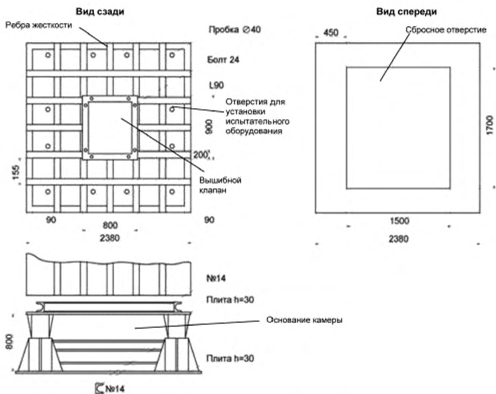
Рисунок А.1 — Схема испытательной взрывной камеры
