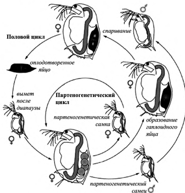
Рисунок В.1 — Цикл развития Daphnia magna Straus
