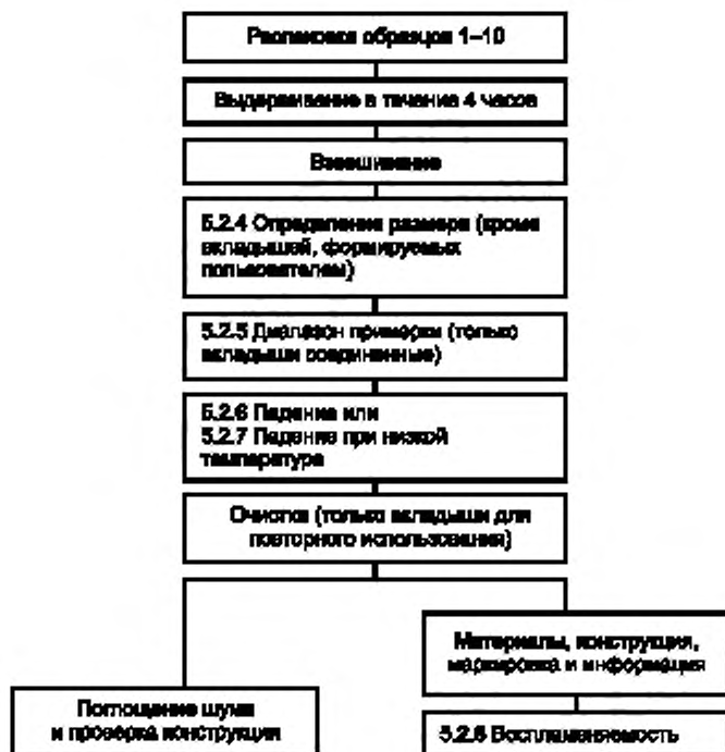
Рисунок В.3 — Блок-схема испытания вкладышей
