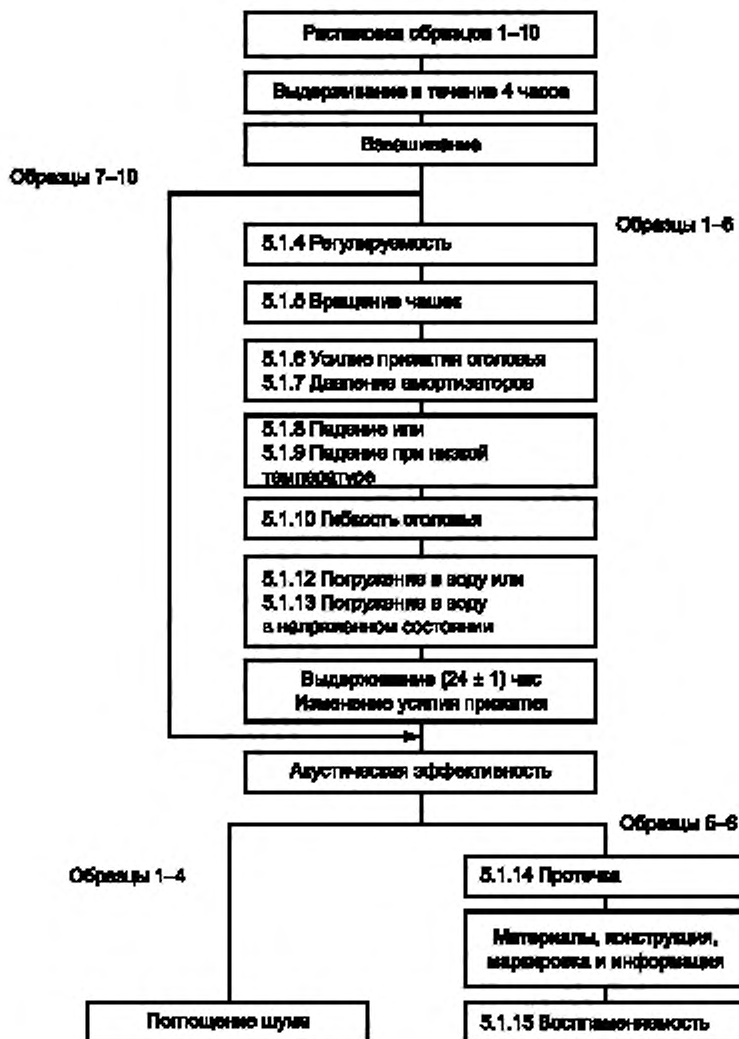
Рисунок В.1 — Блок-схема испытаний наушников с оголовьем
