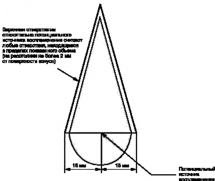
Рисунок 45 — Верхние отверстия
