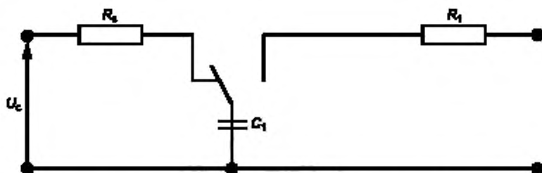
Рисунок D.2 — Испытательный генератор для интерфейса антенны
