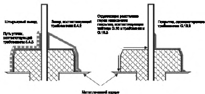
Рисунок O.11 — Покрытие выводов
