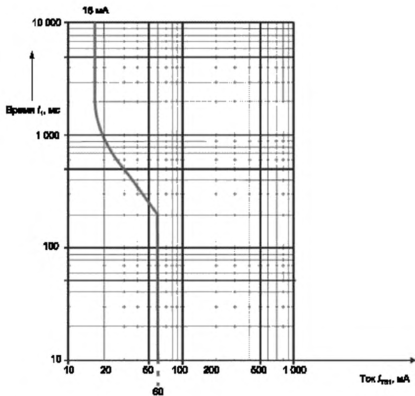
Рисунок Н.2 — Кривая предельно допустимого значения тока I_{TS1} для вызывного сигнала с каднцией
