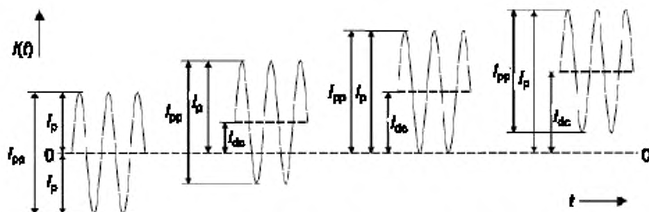
Рисунок N.3 — Пиковое значение тока и удвоенная амплитуда тока
