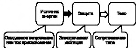
Рисунок 4 — Модель защиты от боли или травм, вызываемых воздействием электричества
