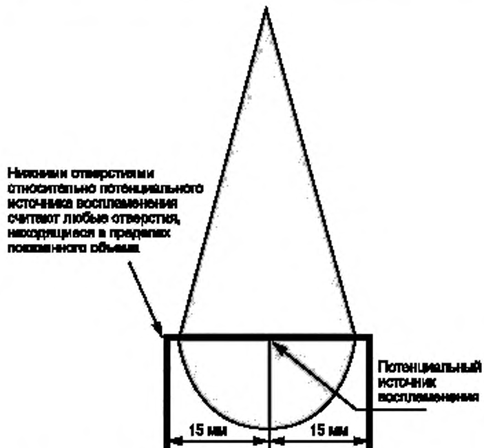
Рисунок 46 — Нижние отверстия
