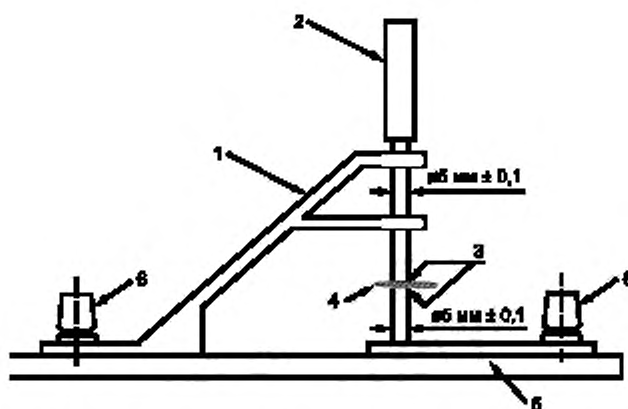
1 — металлическая рама, удерживающая штырь в вертикальном положении (штырь свободно движется в вертикальном направлении); 2 — металлический штырь массой 100 \pm 5 г; 3 — кромки штыря скруглены радиусом 0,5 мм; 4 — испытательный образец; 5 — изоляционное основание; 6 — клеммы для подачи испытательного напряжения
