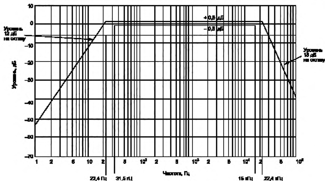
Рисунок Е.1 — Полосовый фильтр для измерения широкополосного шума
