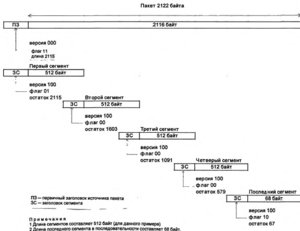
Рисунок 6 — Пример сегментации пакета по источникам данных
