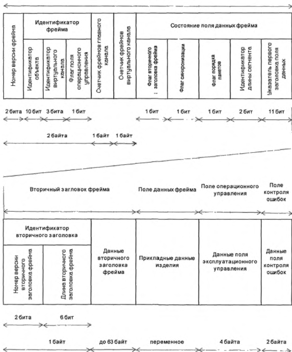
Рисунок 9 — Структура фрейма передачи
