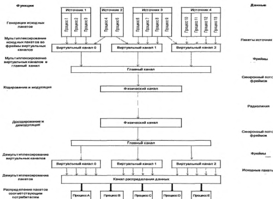
Рисунок 3 — Пример потока телеметрических данных
