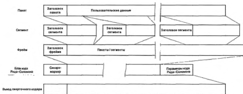
Рисунок 2 — Структуры телеметрических данных
