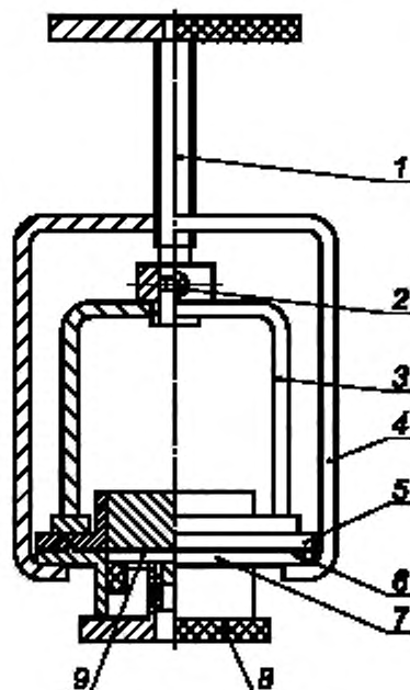
Рисунок 1 — Прибор для испытания образцов изолирующих материалов
