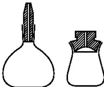
Рисунок 1 — Пикнометры
