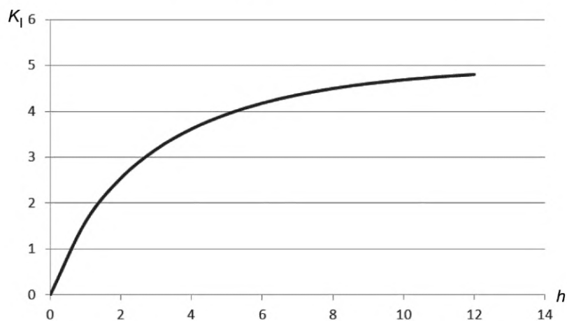
Рисунок А.2 — Зависимость K_1 , дБ, от h , дБ
