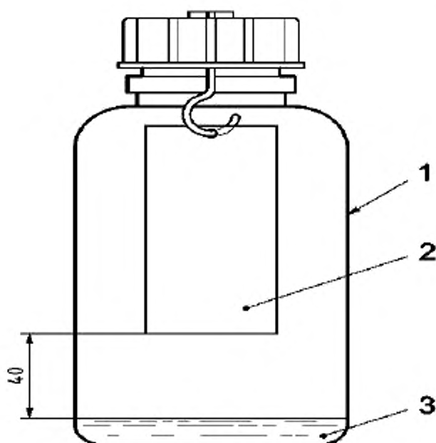
1 – сосуд из полиэтилена; 2 – образец; 3 – вода
