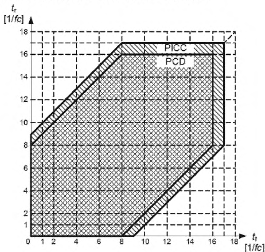
Рисунок 18– Параметры синхронизации модулированного колебательного сигнала типа В
