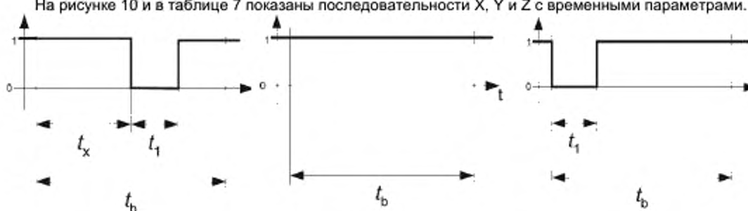
Рисунок 10 – Последовательности для передачи типа A от PCD к PICC
