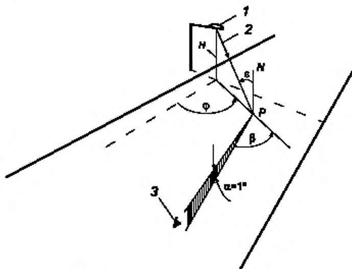
1 — ОП; 2 — луч света в расчетную точку P; 3 — глаз наблюдателя; H — высота светового центра ОП над поверхностью дороги; N — нормаль к поверхности дороги в точке P; \beta — угол отклонения; \alpha — угол падения света; \alpha — угол наблюдения; \varphi — азимутальный угол точки P
