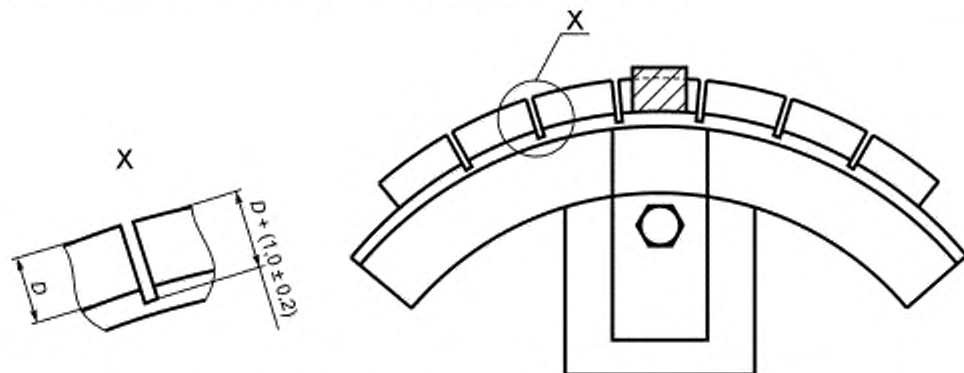
Рисунок 1 — Колодка с накладкой, разделенная на сегменты
