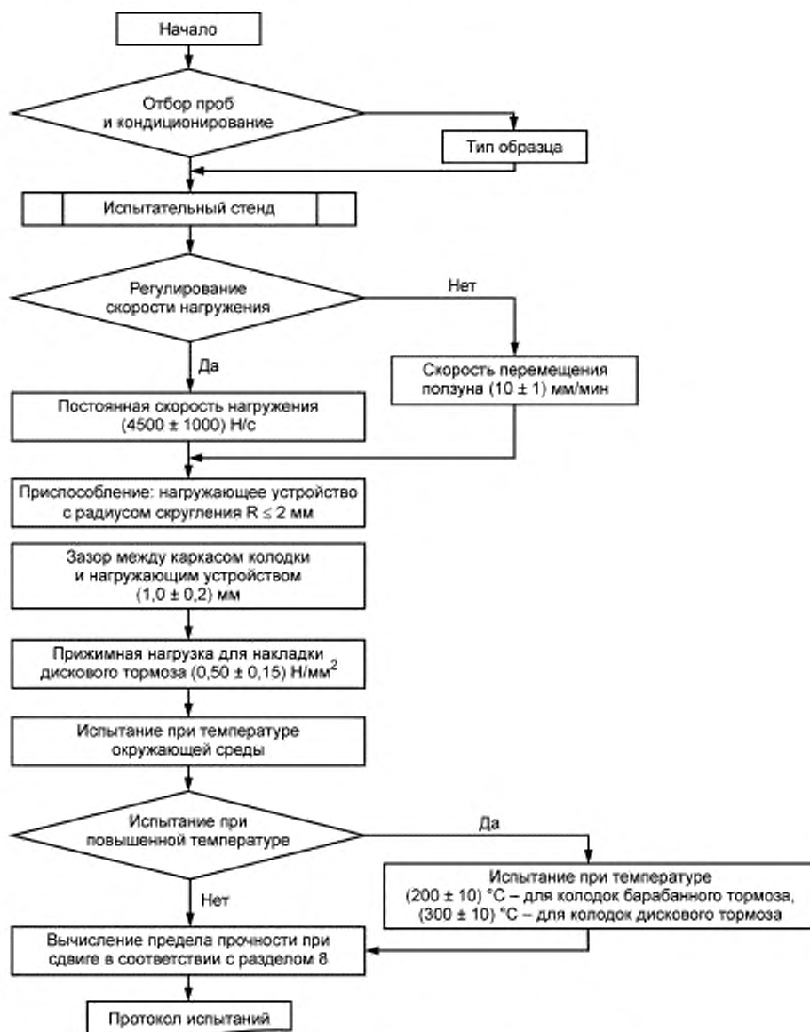
Рисунок А.1 — Блок-схема проведения испытаний
