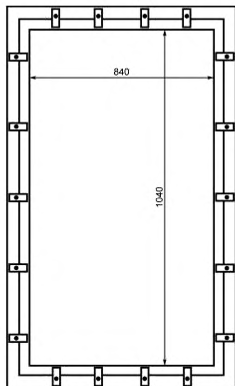
Рисунок В.2 — Наружная рама
