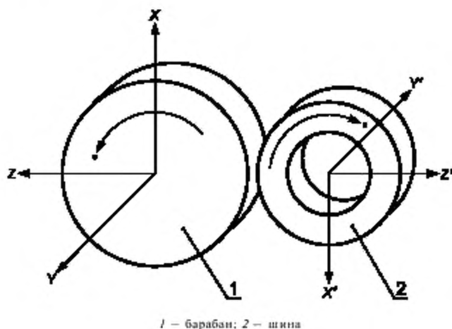
Рисунок 1 — Система базисных осей для сил
