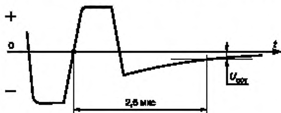
Рисунок 9 — Симметрия сигнала
