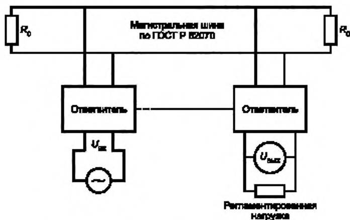
Рисунок 5 — Измерение затухания в магистральной шине/ответвителе
